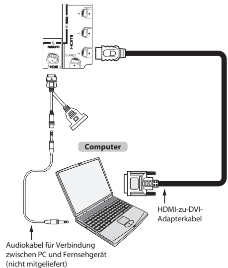
Rückseite des Fernsehgeräts
