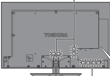
Kabelklammern (für Wandhalterung-Typ)
